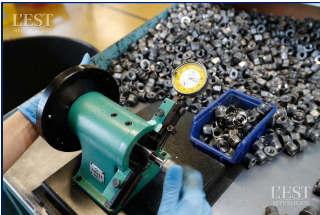
Tri et vérification de pièces mécaniques dans les ateliers de la société Adapt'Performance à Morvillars
